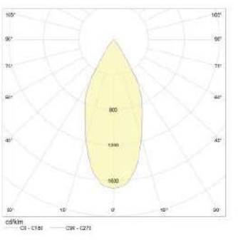
45° Reflector
