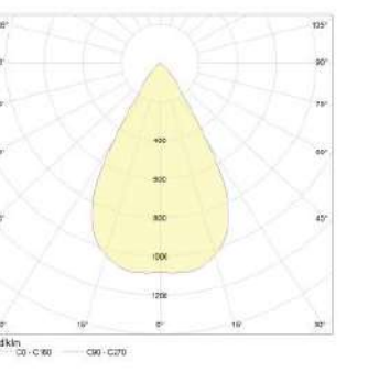
60° Reflector
