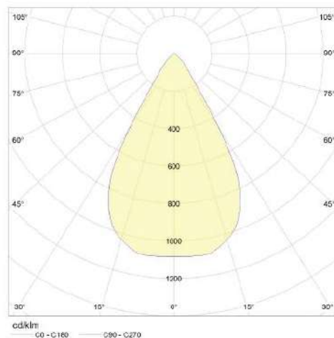
60° Reflector
