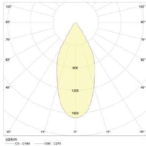
45° Reflector
