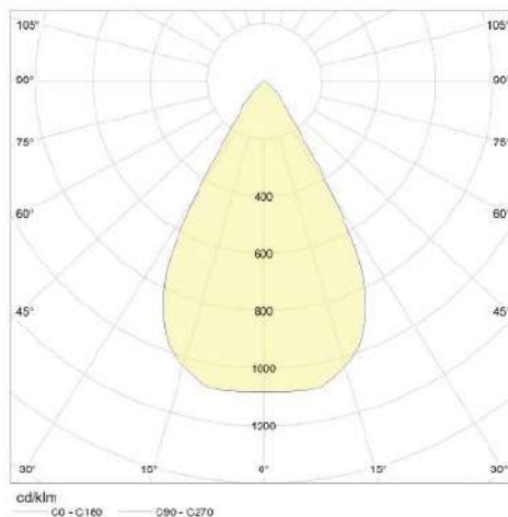
60° Reflector
