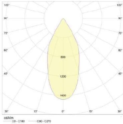
45° Reflector
