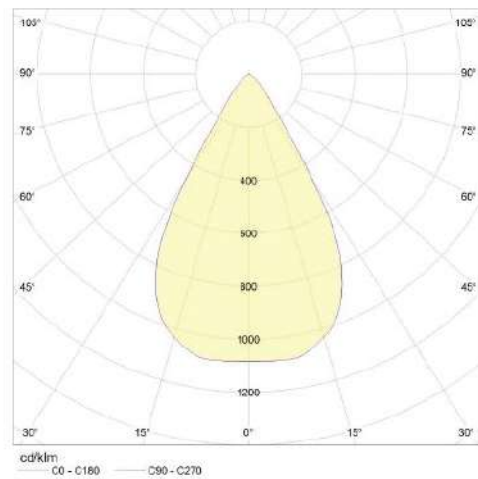
60° Reflector
