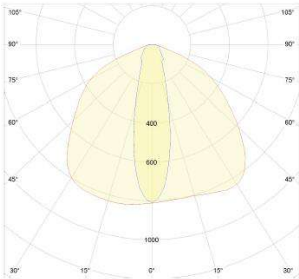
31°+119° Lens
