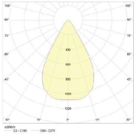
60° Reflector
