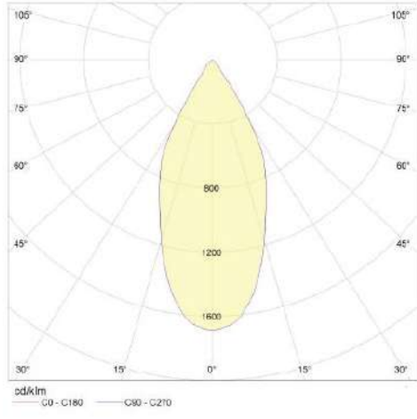
45° Reflector
