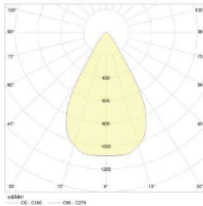
60° Reflector
