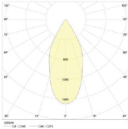
45° Reflector
