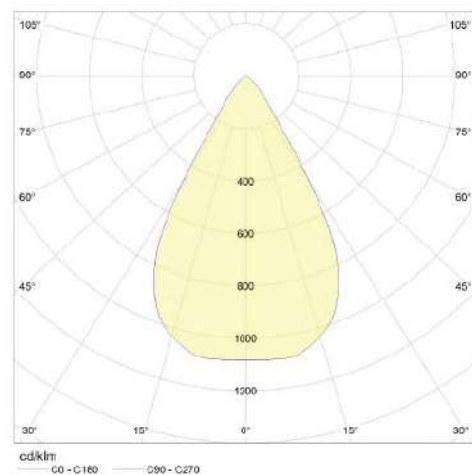
60° Reflector
