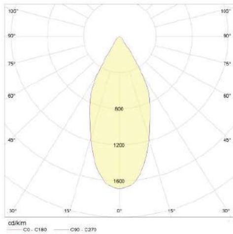
45° Reflector
